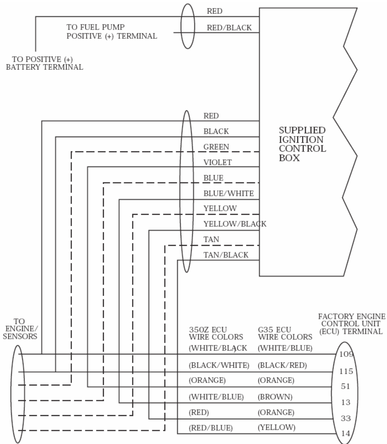
Fig. 10-d / Wiring Diagram
